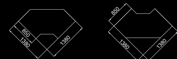
850mm 宽, E6 内角柜
