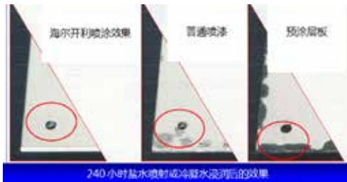
盐雾试验结果
