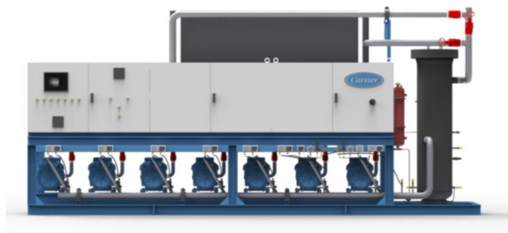
覆叠CO2机组
