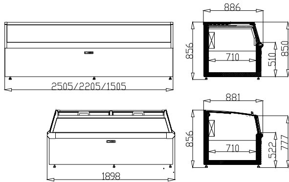
玲珑系列组合式整机冷冻柜
